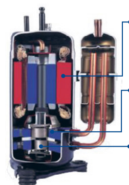
Двухроторный инверторный компрессор
