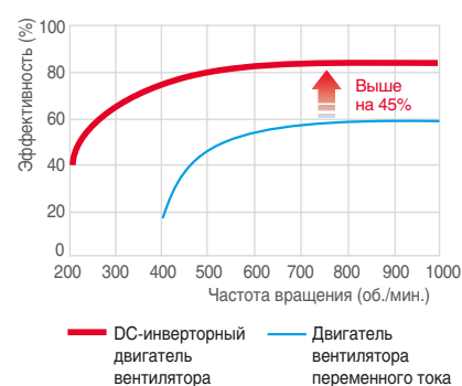
DC-инверторный двигатель вентилятора
